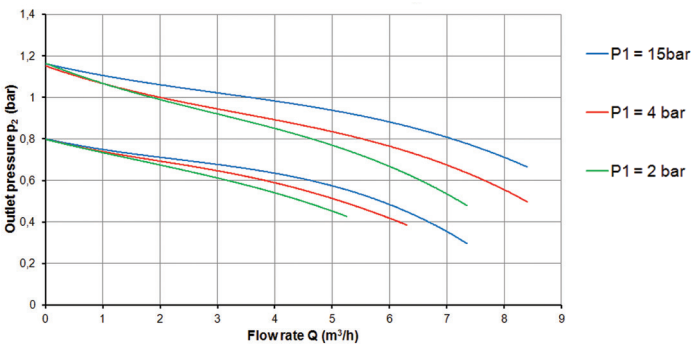
Acetylene 25/1,5 bar
