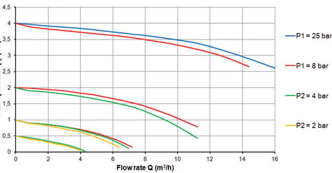
Propane 25/ 4 bar
