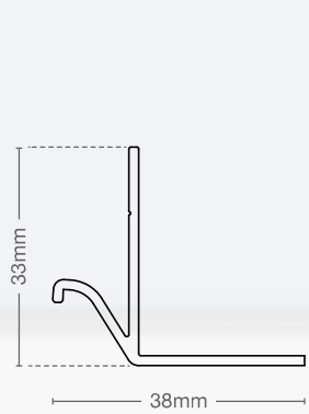
Starter bar CL 001BK
