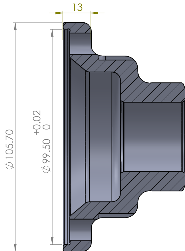
SECTION A-A SCALE 1 : 1
